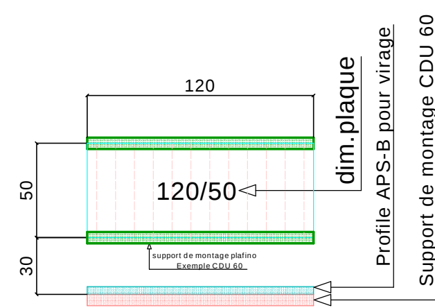
Plaque de pose ONIVO Plafino
