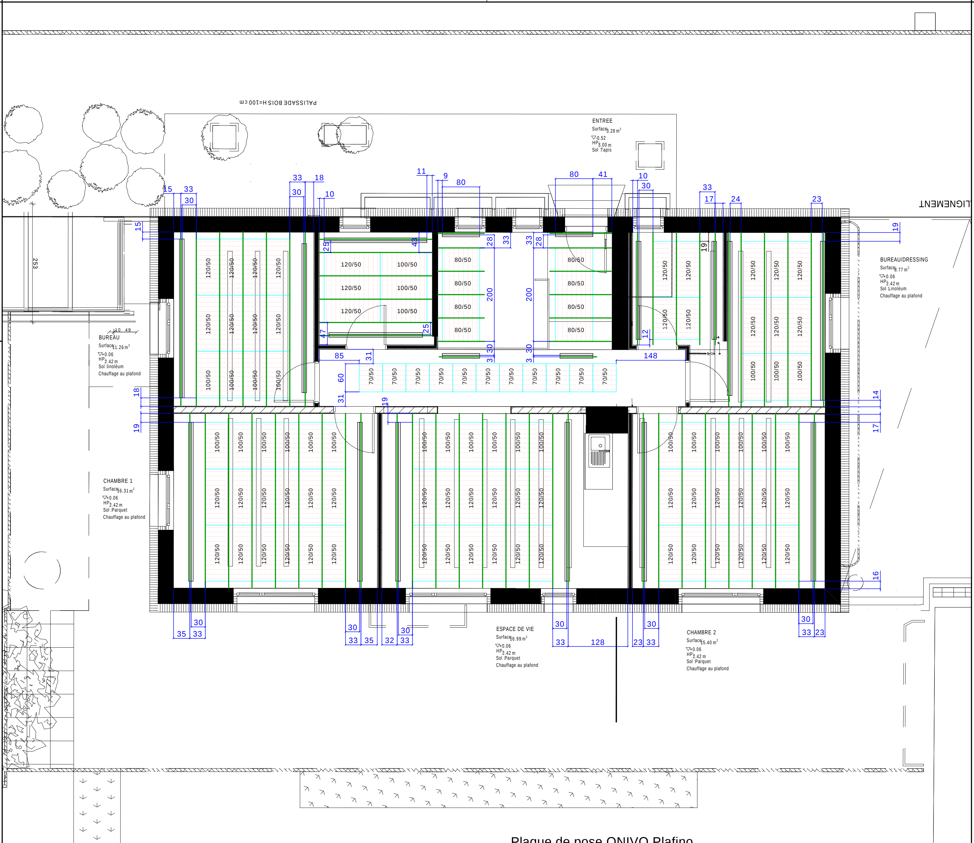
Plaque de pose ONIVO Plafino
